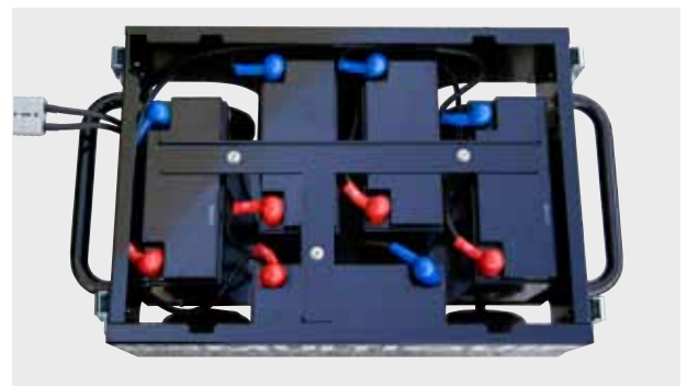
El compartimento de la batería almacena cinco baterías recargables de 12 voltios.
